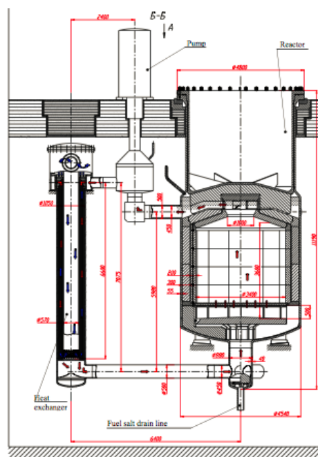
Figure 13 : Vue en coupe du projet MOSART
