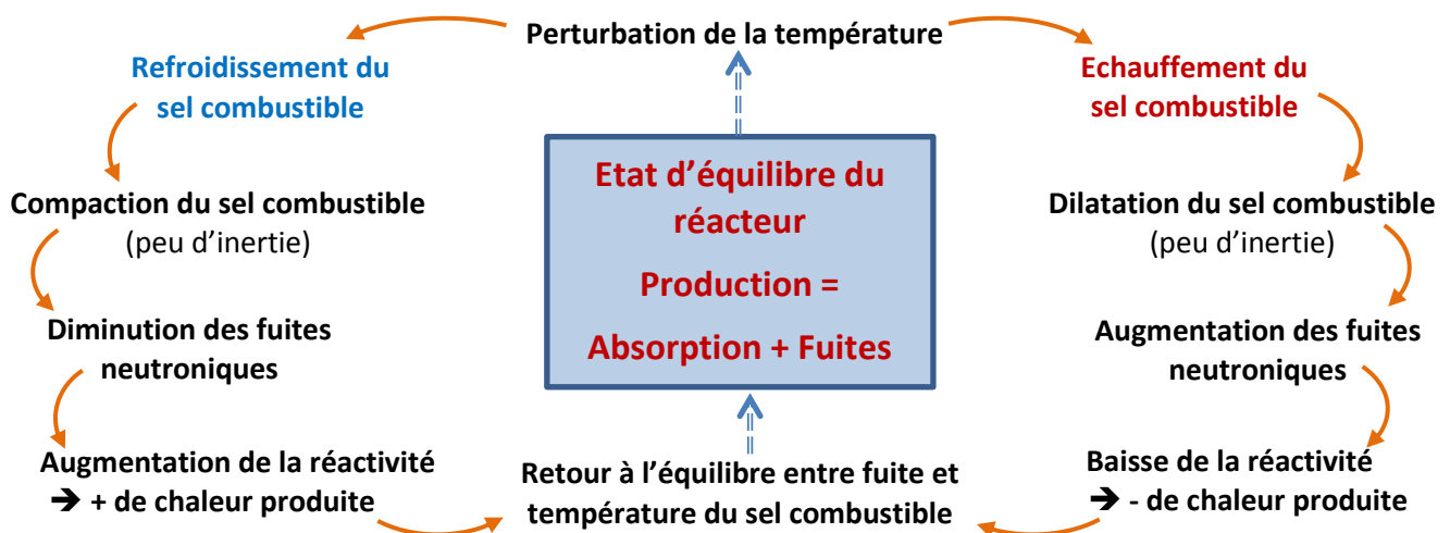
Figure 26 : Boucle de contre-réaction des réacteurs à combustible liquide garantissant le retour à l'équilibre neutronique et permettant le pilotage de la puissance.
