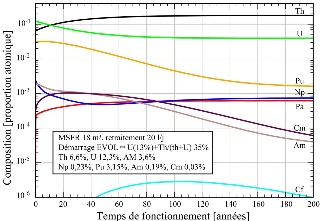
Figure 32 : Exemple de calcul d'incinération à partir d'un chargement initial du projet EVOL
