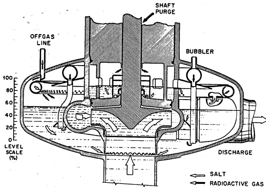
Figure 7 : Pompe primaire du MSRE.
