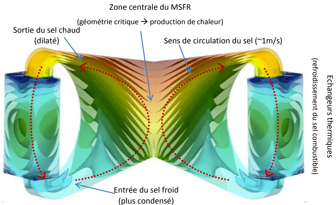
Figure 28 : Carte de températures du sel dans une vue en coupe de deux secteurs du circuit combustible du MSFR : échauffement dans la zone centrale, refroidissement dans les échangeurs.
