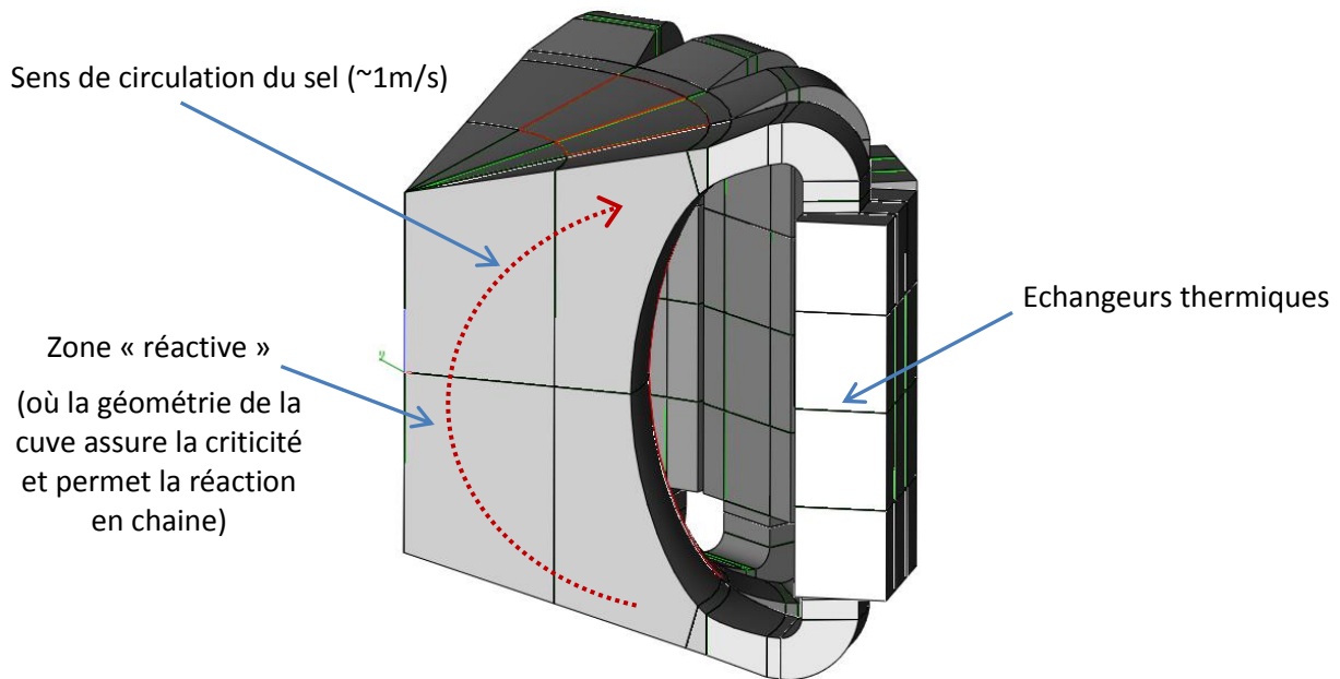
Figure 29 : Vue de plusieurs secteurs (échangeurs +pompes) immergés dans la cuve du MSFR
