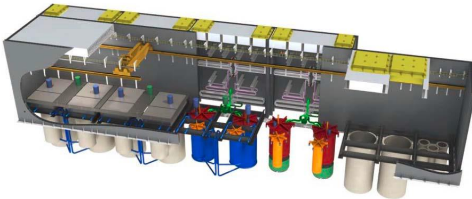
Figure 19 : vue de Thorcon
