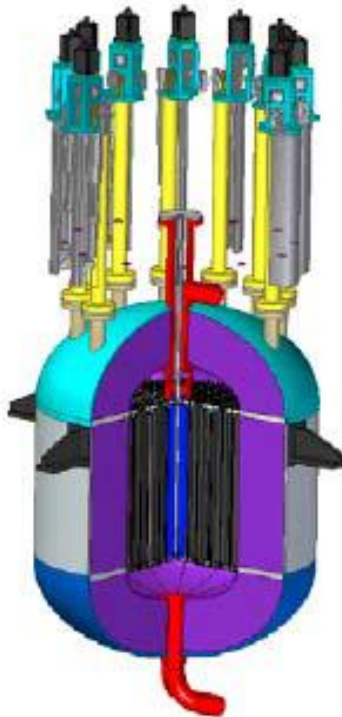
Figure 11 : Vue du bloc réacteur
