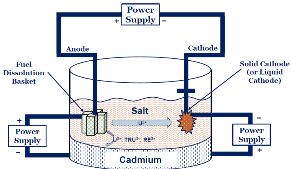
Figure 34 : Schéma de principe des extractions par pyrochimie
