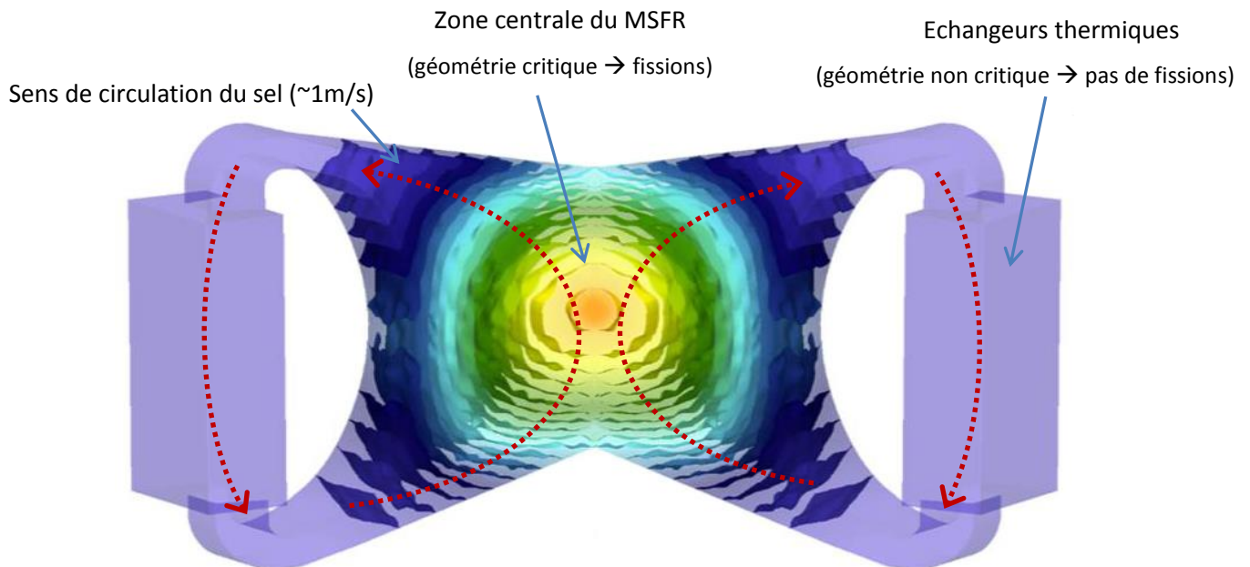
Figure 27 : Répartition du taux de fission dans une vue en coupe de deux secteurs du circuit combustible du MSFR : la zone centrale permet la réaction en chaîne du fait de la géométrie critique, dans les échangeurs la géométrie ne permet plus la réaction en chaîne.
