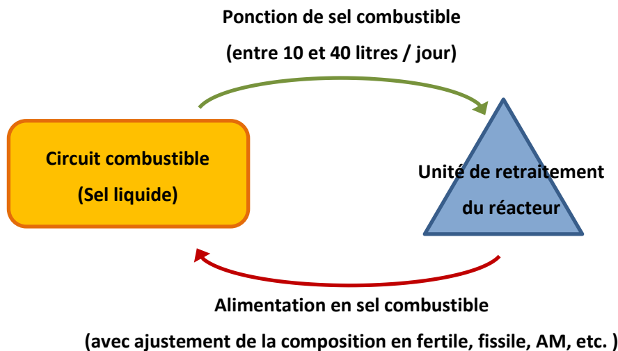
Figure 33 : Schéma de principe du retraitement du sel combustible par l'unité au sein du réacteur
