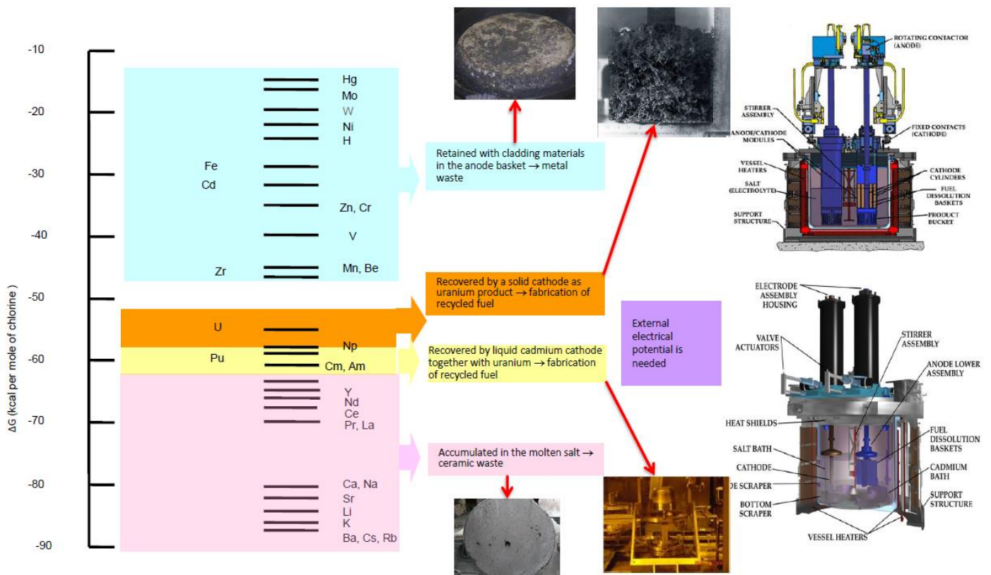
Figure 36 : Principe du procédé de séparation par électro chimie utilisé ou proposé pour les combustibles métalliques (EBR2)
