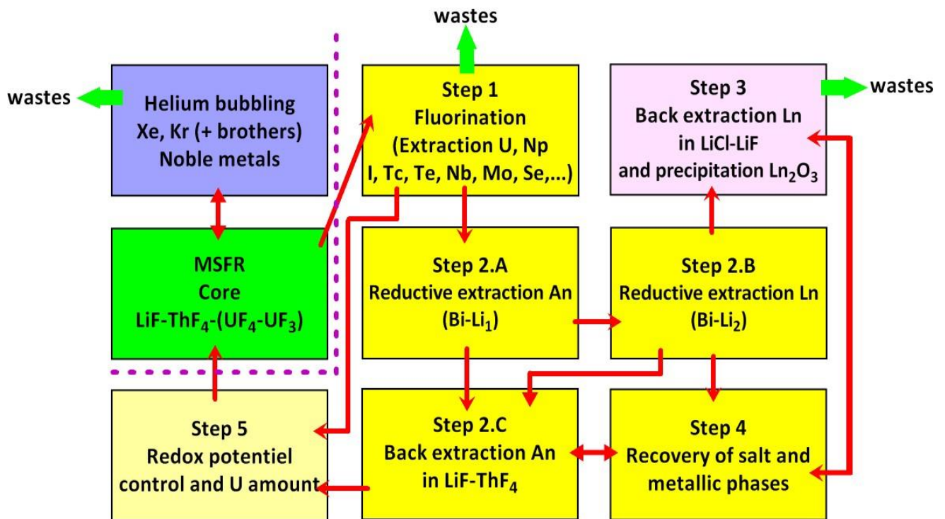
Figure 35 : Etapes possibles pour un retraitement du sel combustible d'un MSR
