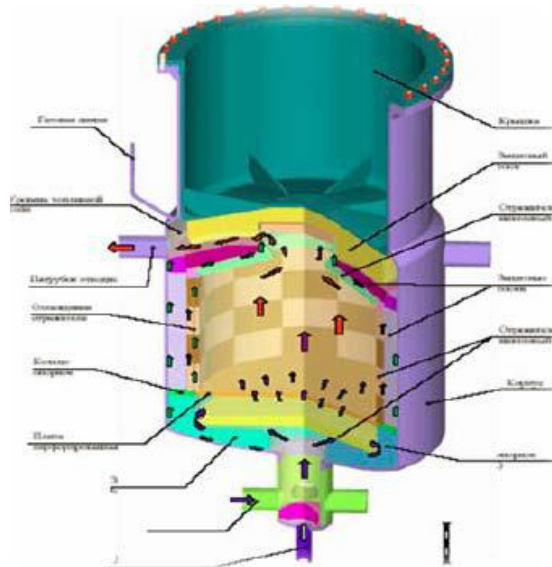
Figure 12 : Vue du bloc réacteur MOSART
