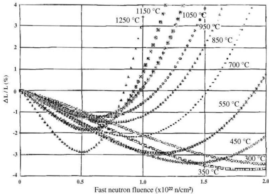
Figure 24 : Variation dimensionnelle du graphite en fonction de la fluence et de la température.
