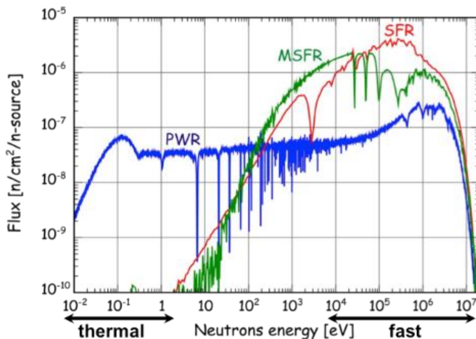
Figure 31 : Spectre neutronique du MSFR (courbe verte)
