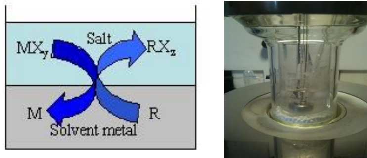
Figure 37 : Schéma de principe d'un procédé d'extraction réductrice sur métal fondu (ici bismuth liquide)
