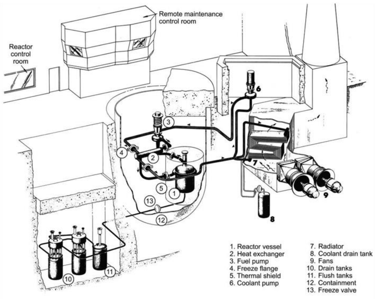
Figure 3 : Vue générale du MSRE.
