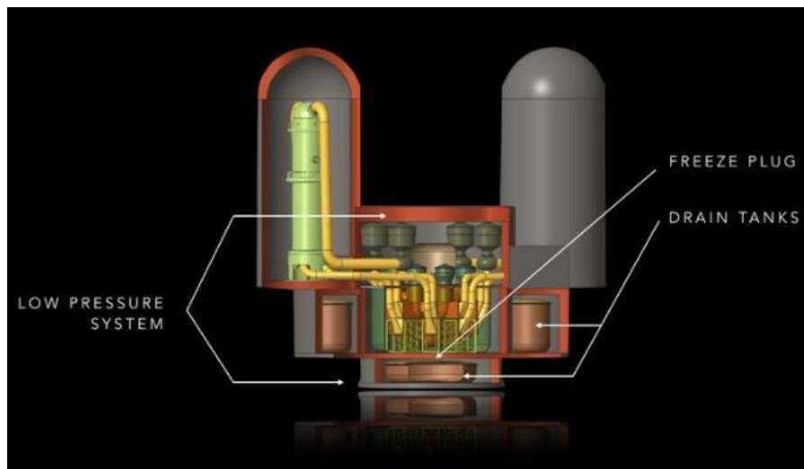
Figure 17 : Le MCSFR d'Elysium Industry
